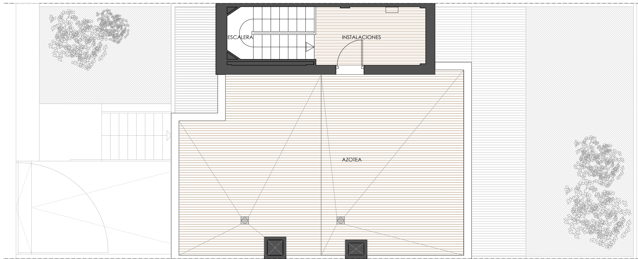
PLANTA CAJETÓN. TIPO 01'
