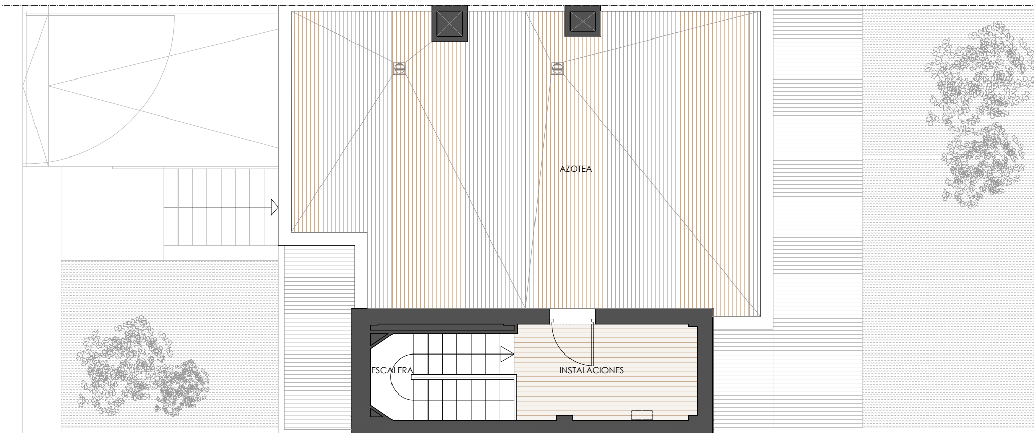
PLANTA CASETÓN. TIPO 02-B'
