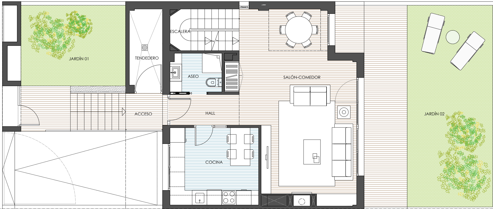
PLANTA BAJA. TIPO 02-A'
