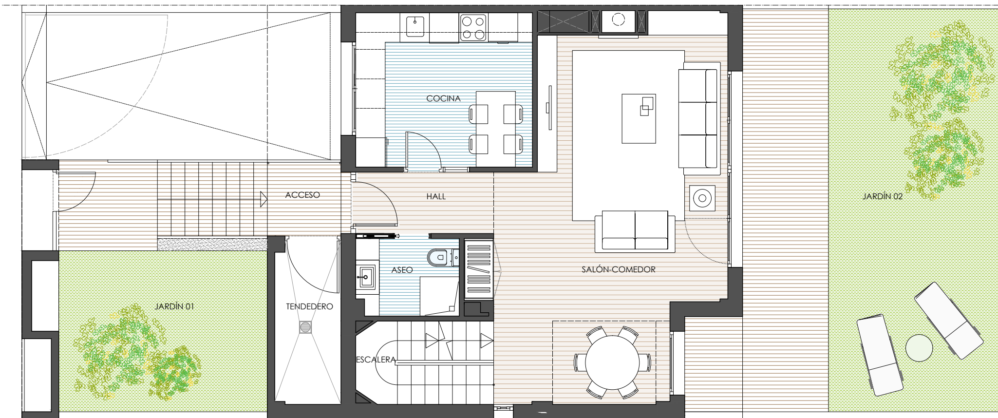
PLANTA BAJA. TIPO 02-A
