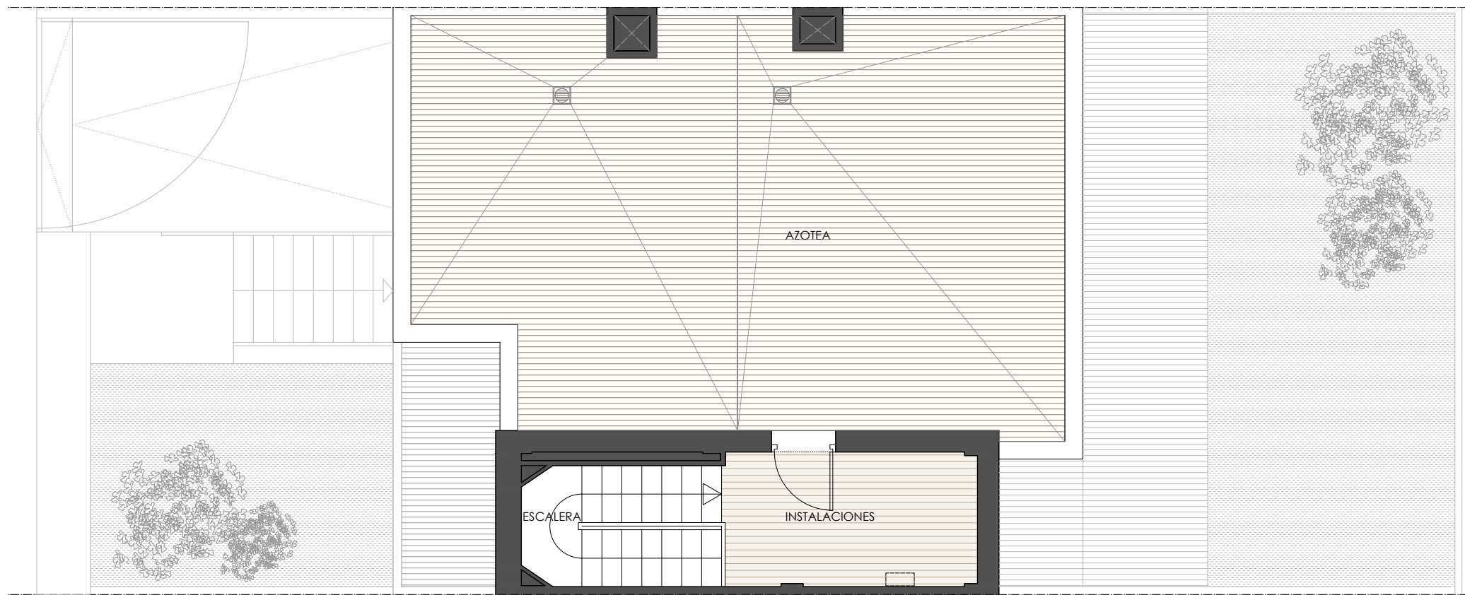
PLANTA CASETÓN. TIPO 01
