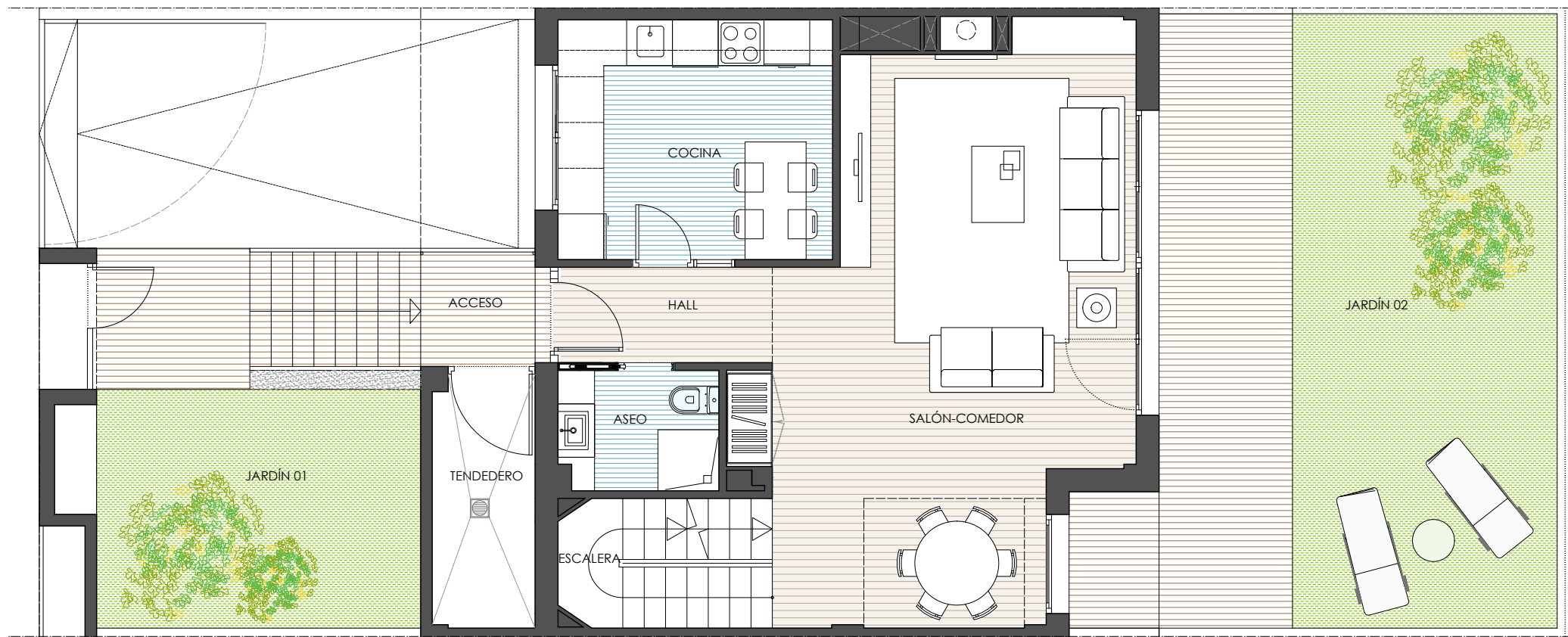
PLANTA BAJA. TIPO 01
